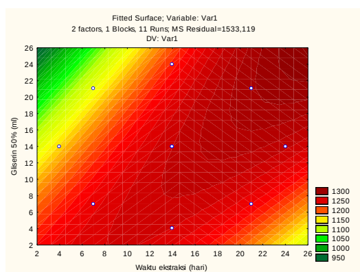
Gambar 9. Kontur optimasi 2
