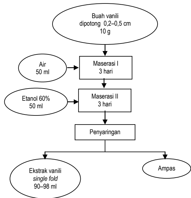
Gambar 2. Maserasi 2 tahap 1 kali penyaringan
