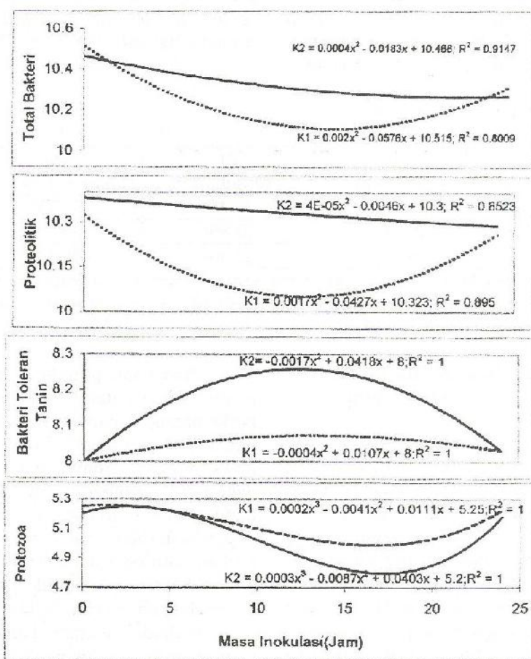
Grafik 1. Dinamika Populasi Mikroba Rumen
