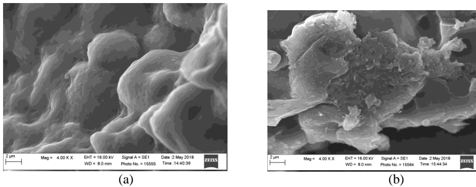
Gambar 4. Morfologi nanopartikel tapioka terhidrolisis (a)2 jam dan (b) 24 jam pada perbesaran 4000 kali
