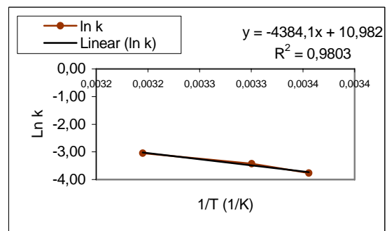
Gambar 5. Kurva hubungan antara 1/T dengan ln k pada bubuk jahe merah tanpa bahan pengisi
