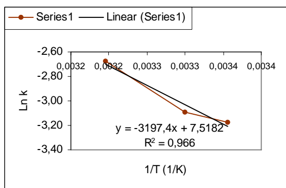
Gambar 6. Kurva hubungan antara 1/T dengan ln k pada bubuk jahe merah dengan bahan pengisi sukrosa 20 %
