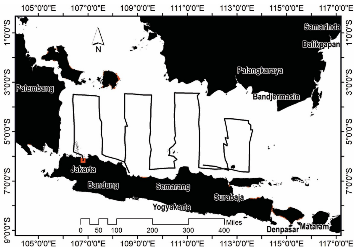
Gambar 1. Jalur transek hidroakustik untuk estimasi sumberdaya ikan.
