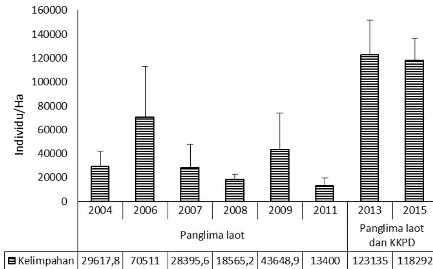
Gambar 10. Kondisi kelimpahan ikan karang per tahun (Sumber: Olahan data primer dan sekunder).
