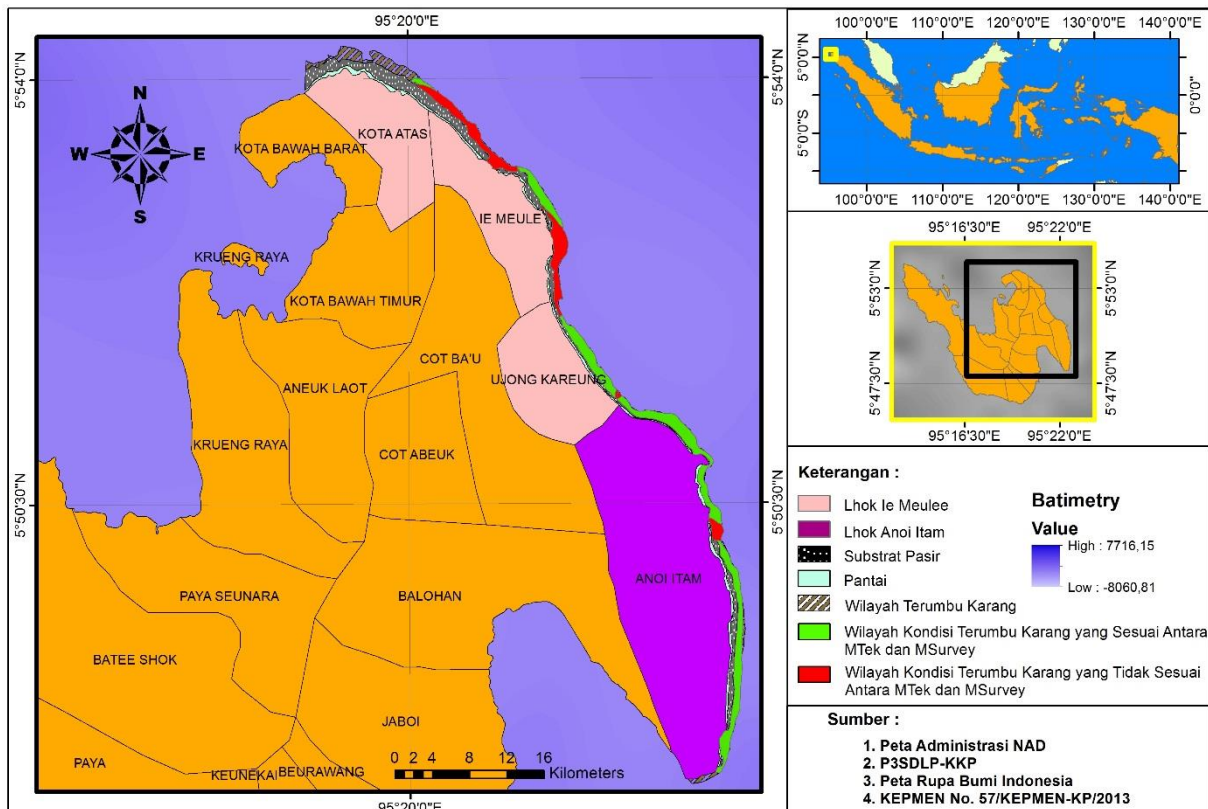
Gambar 5. Overlay pemetaan PEL dan survei kondisi terumbu karang.
