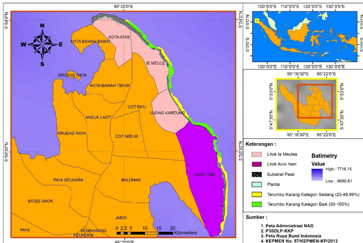
Gambar 4. Mapping survei kondisi terumbu karang.
