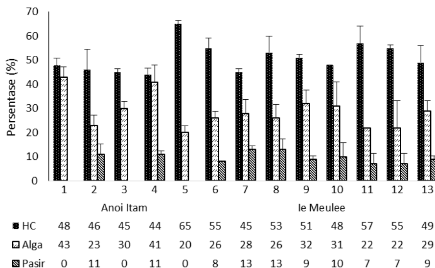
Gambar 3. Persentase penutupan karang hidup, alga dan pasir.
