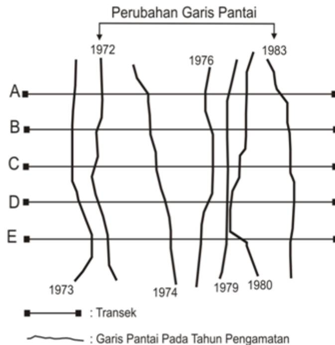
Gambar 2. Ilustrasi perhitungan menggunakan program Digital Shoreline Analysis System .
