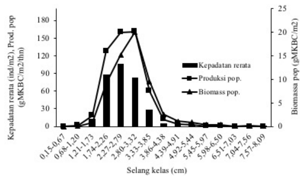
Gambar 7. Kepadatan rata-rata, estimasi produksi dan biomassa tahunan pada setiap kelas ukuran berbeda B. violacea var. celebensis di muara Sungai Lasolo.
