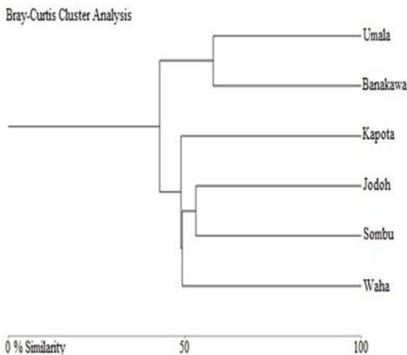
Gambar 2. Dendrogram berdasarkan kesamaan spesies setiap lokasi.
