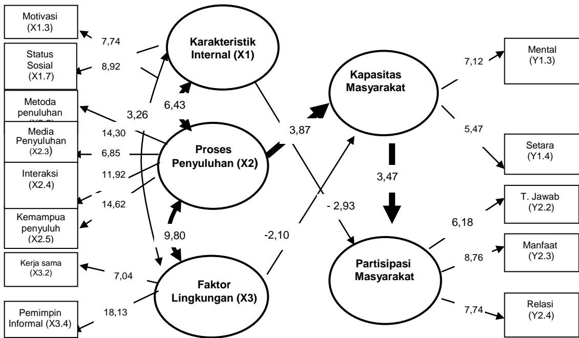
Gambar 2 Statistik t -hitung parameter model struktural partisipasi
