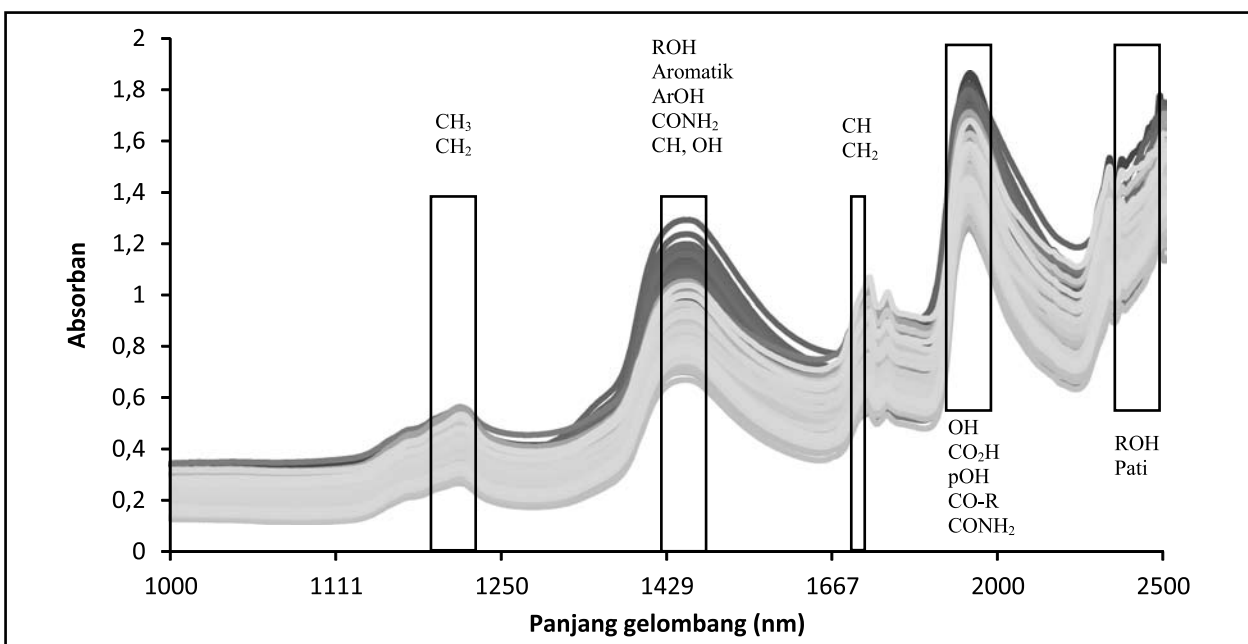
Gambar 3. Spektrum absorban NIR kelapa sawit.
