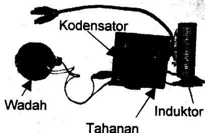
Gambar 7. Rangkaian LRC.
