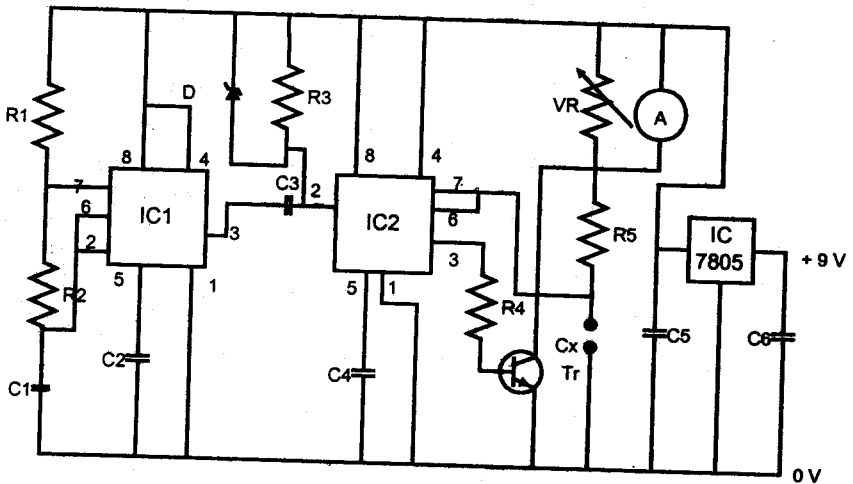
Gambar 6. Skema Alat ukur kapasitansi
