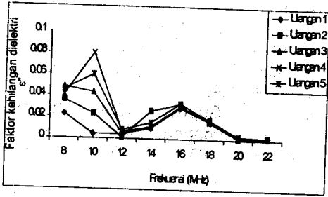
Gambar 13. Grafik pengaruh frekuensi terhadap nilai faktor kehilangan dielektrik ( \epsilon'' ) lada pada kadar air 19,18 %
