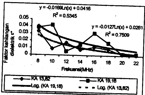
Gambar 15. Grafik pengaruh frekuensi terhadap rata-rata nilai faktor kehilangan dielektrik ( \epsilon'' ) lada.
