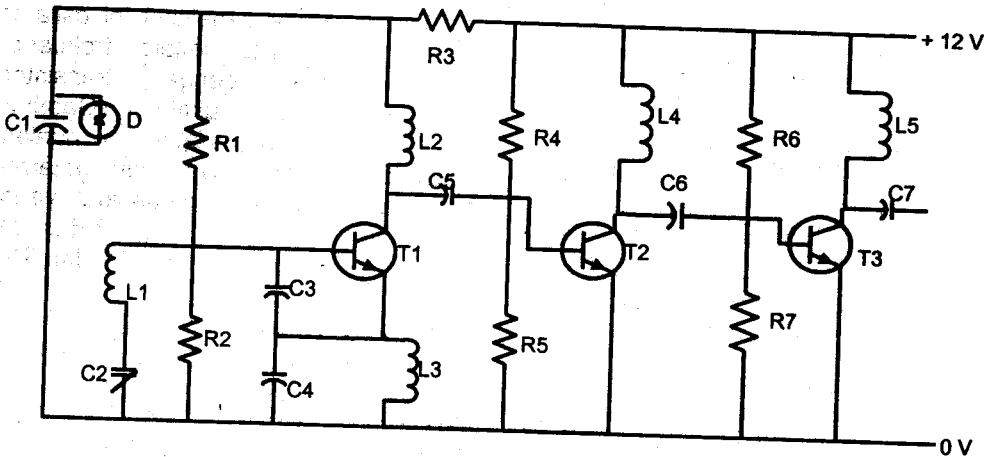
Gambar 5. Rangkaian elektronik untuk membangkitkan gelombang radio.
