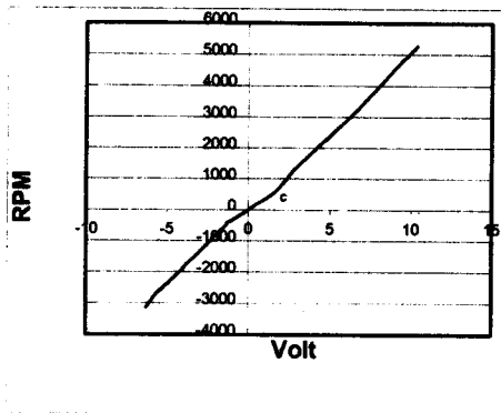
Gambar 8. Grafik hubungan tegangan kerja dan rpm motor pada pencatuan 12 Volt
