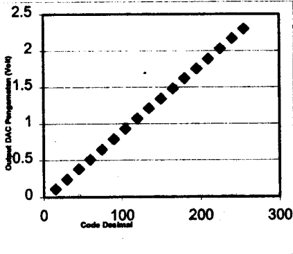
Gambar 5. Hubungan set desimal dan tegangan Keluaran DAC
