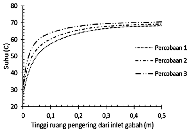
Gambar 7. Suhu gabah daerah spout .
