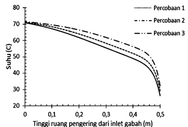
Gambar 8. Suhu gabah daerah downcomer .
