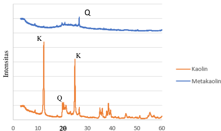
Gambar 3. Pola difraksi sinar-X metakaolin
