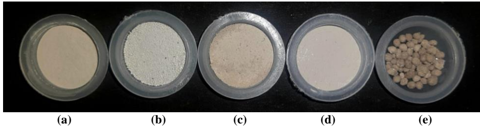
Gambar 4. Sampel (a) zeolit alam serbuk (b) geopolimer serbuk (c) komposit zeolit-geopolimer granul kecil (serbuk) (d) zeolit + geopolimer ( physical mixing ) (e) komposit zeolit-geopolimer granul besar
