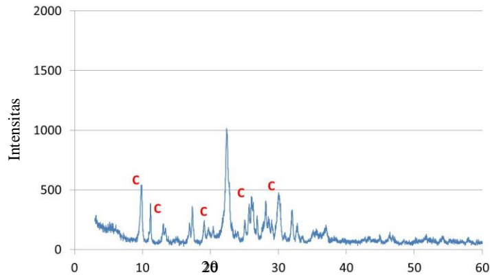
Gambar 1. Pola difraksi sinar-X zeolit alam Nanggung
