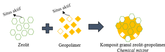
Gambar 6. Mekanisme pembentukan komposit granul zeolit-geopolimer
