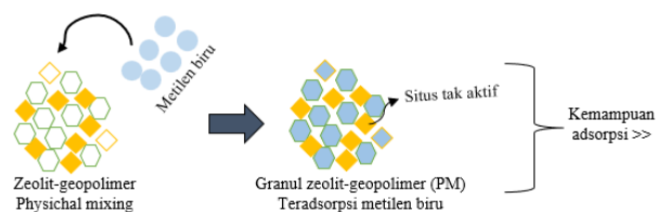
Gambar 13. Mekanisme adsorpsi metilen biru pada zeolit + geopolimer (PM)
