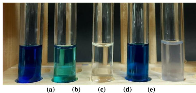
Gambar 9. Hasil pengaliran (a) metilen biru 25 ppm pada sampel (b) zeolit alam granul, (c) zeolit alam serbuk, (d) komposit zeolit-geopolimer granul besar, dan (e) komposit zeolit-geopolimer granul besar
