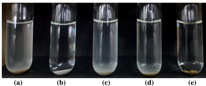
Gambar 14. Uji ketahanan sampel (a) zeolit alam serbuk (b) geopolimer serbuk (c) zeolit + geopolimer ( physical mixing ) (d) komposit zeolit-geopolimer granul kecil (serbuk) (e) komposit zeolit-geopolimer granul besar dalam air
