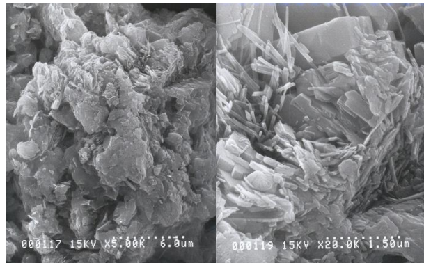
Gambar 2. Foto SEM zeolit alam Nanggung
