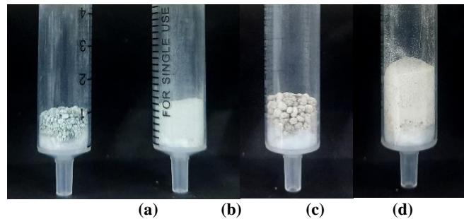
Gambar 8. Sampel (a) zeolit alam granul, (b) zeolit alam serbuk, (c) komposit zeolit-geopolimer granul besar, dan (d) komposit zeolit-geopolimer granul kecil (serbuk) pada simulasi filter pengolahan limbah pewarna
