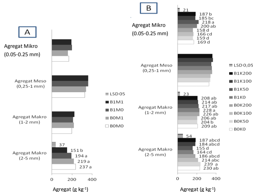
Gambar 1. Pengaruh interaksi (A) B. decumbens dan mikoriza dan (B) Brachiari decumbens dan kompos jerami diperkaya K terhadap makroagregat 2-5 mm (makro 1), makroagregat 1-2 mm (makro 2), meso agregat (0.25-1 mm) dan mikro agregat (0.05-0.25 mm). Label data pada parameter yang sama diikuti huruf kecil yang sama, tidak berbeda nyata pada taraf nyata 10% menurut LSD.
