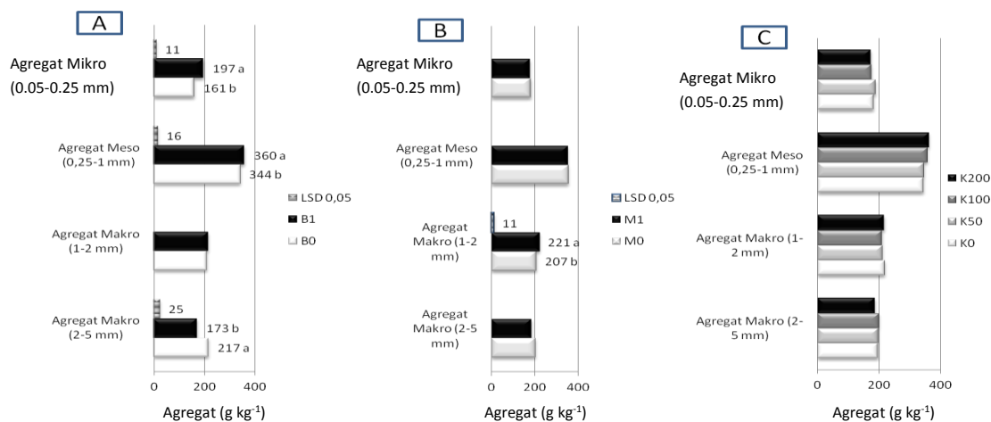
Gambar 2. Pengaruh B. decumbens (A), mikoriza (B) dan kompos jerami diperkaya K (C) terhadap stabilitas agregat ( \text{g kg}^{-1} ) dari makroagregat 1 (2-5 mm), makroagregat 2 (1-2mm), mesoagregat (0.25-1 mm) dan mikroagregat (0.05-0.25 mm). Label data pada parameter yang sama, diikuti oleh huruf kecil yang sama, tidak berbeda nyata pada taraf nyata 5% menurut LSD.
