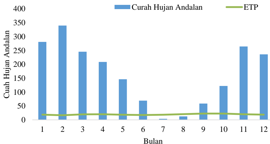
Gambar 2 Nilai CH andalan Kecamatan Cibinong peluang 80% dan ETP
