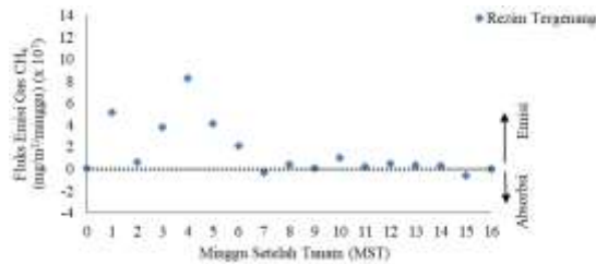
Gambar 2 Fluks gas CH 4 rezim tergenang selama satu musim tanam.
