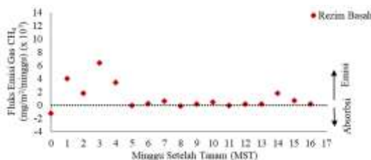
Gambar 3 Fluks gas CH 4 rezim basah selama satu musim tanam.
