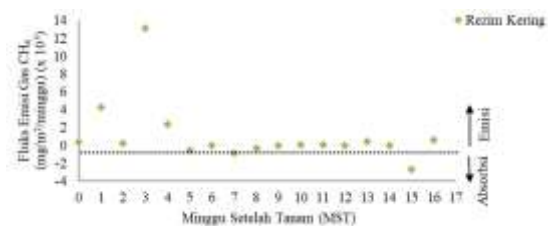
Gambar 4 Fluks gas CH 4 rezim kering selama satu musim tanam.
