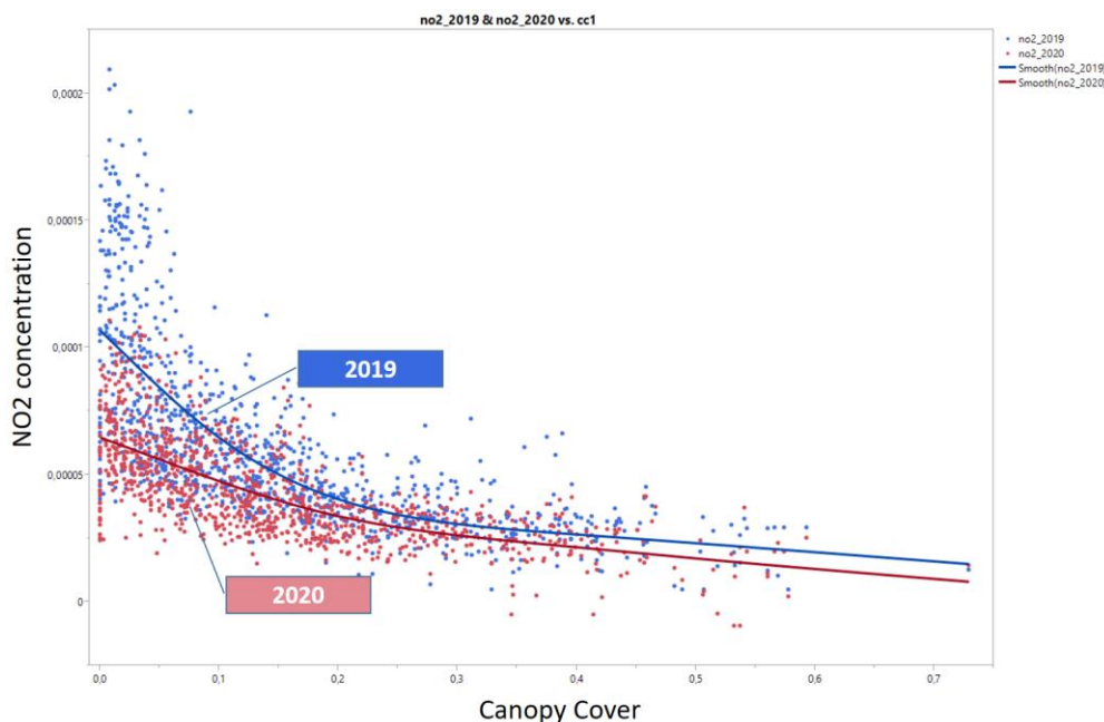
Gambar 11 Korelasi tutupan tajuk dan konsentrasi NO 2 tahun 2019 dan 2020
