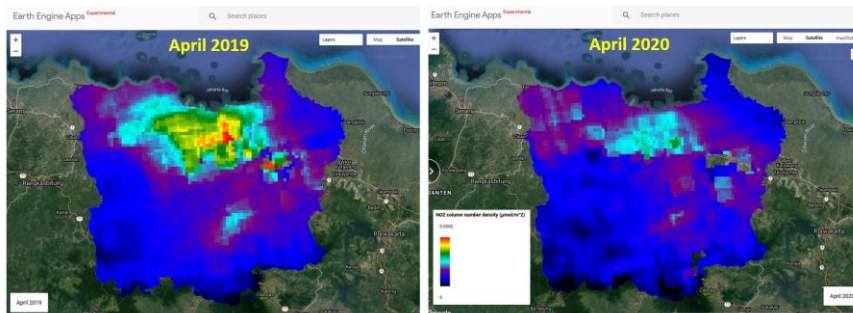
Gambar 4 Perubahan konsentrasi NO 2 di Jabodetabek sebelum adanya pandemi virus Corona (April 2019) dan periode awal terjadinya pandemi (April 2020)
