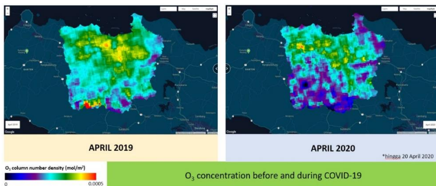
Gambar 5 Perubahan konsentrasi O 3 di Jabodetabek sebelum adanya pandemi virus Corona (April 2019) dan periode awal terjadinya pandemi (April 2020)
