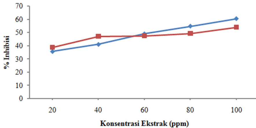
Gambar 1 Kurva aktivitas antioksidan ekstrak Spirulina platensis segar dengan pelarut aseton dan etil asetat berbagai konsentrasi pada panjang gelombang 517 nm dengan menggunakan spektrofotometer UV-Vis
