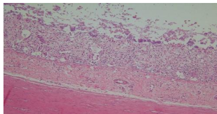
Gambar 3 Erosi vili
