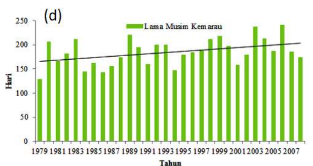
Gambar 5 Pola awal musim kemarau dan hujan di Kapuas pada cluster 1 (a) dan cluster 2 (b) serta lama musim kemarau pada cluster 1 (c) dan cluster 2 (d)
