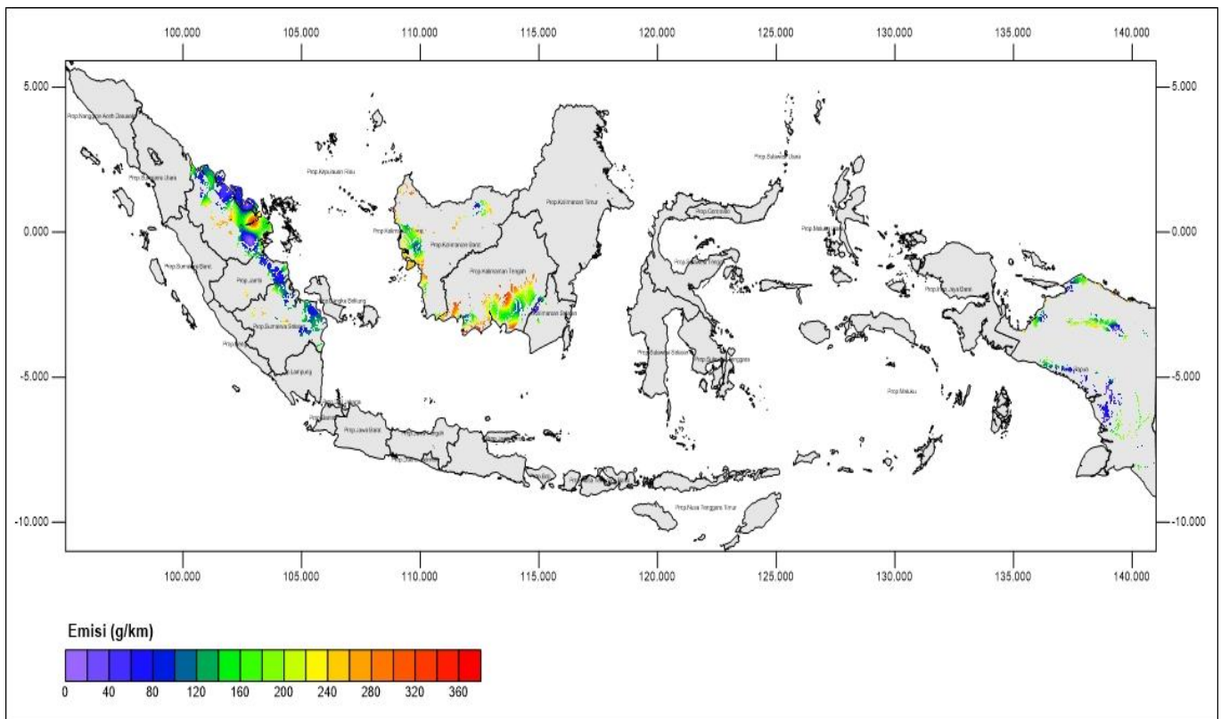
Gambar 4 Peta emisi karbon lahan gambut komposit dari citra SMAP pada bulan Januari 2018. Satuan dinyatakan dalam gram karbon per kilometer persegi
