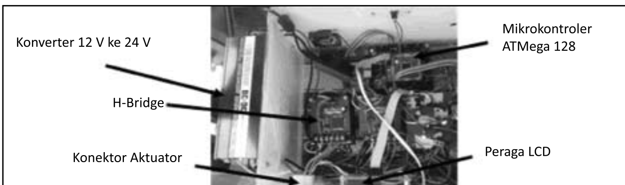
Gambar 6. Rangkaian elektronika pengendali pedal rem dan tuas transmisi
