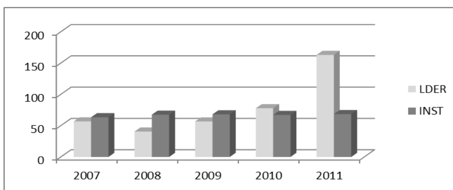
Gambar 3. Pengaruh INST terhadap LDER
