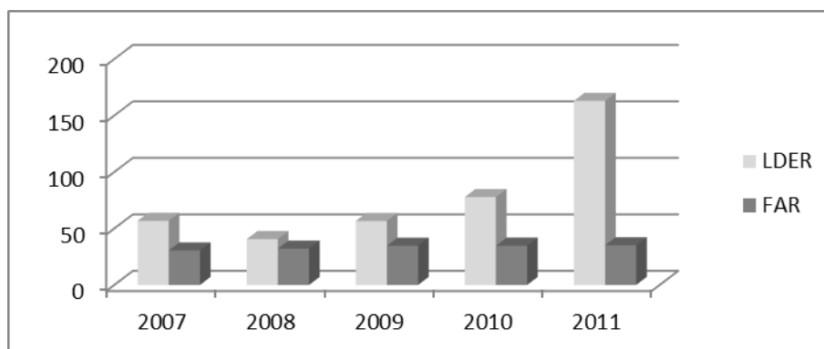
Gambar 4. Pengaruh FAR terhadap LDER
