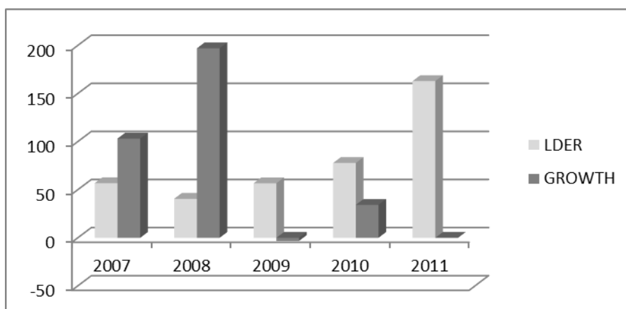
Gambar 6. Pengaruh GROWTH terhadap LDER
