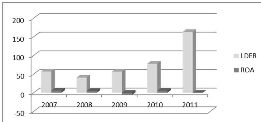
Gambar 5. Pengaruh ROA terhadap LDER
