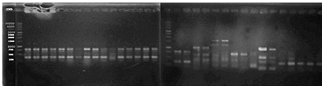
Gambar 1. Elektroforegram hasil amplifikasi DNA 32 aksesori sayuran polong menggunakan primer ISSR kode PKBT 3.No 1-14 = VUu (kacang tunggak); No.15-18 = VUs (kacang panjang); N.19-20 = VS (kacang Bogor); No. 21-22 = PL (koro kratok); No. 23 = PV (kacang merah); No. 24 = CE (koro pedang); No. 25 = GM (kedelai); 26-27 = MP (koro benguk); No. 28-32 = PT (kecipir).
